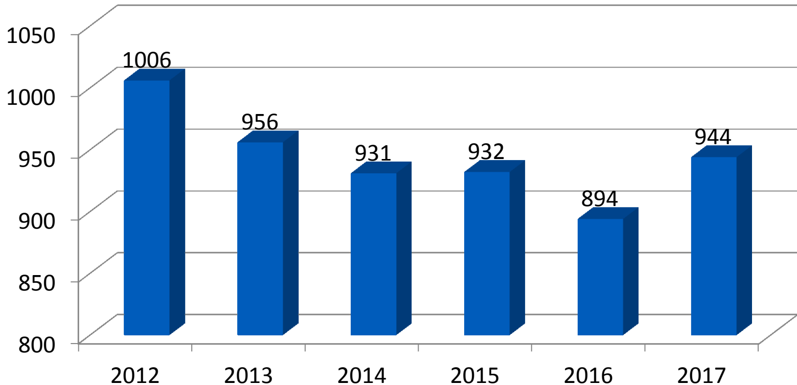
Valid PECs 2012-2017
